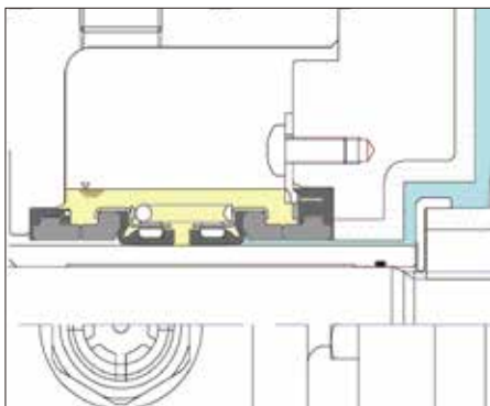
【ダブルメカニカルシール断面図】
