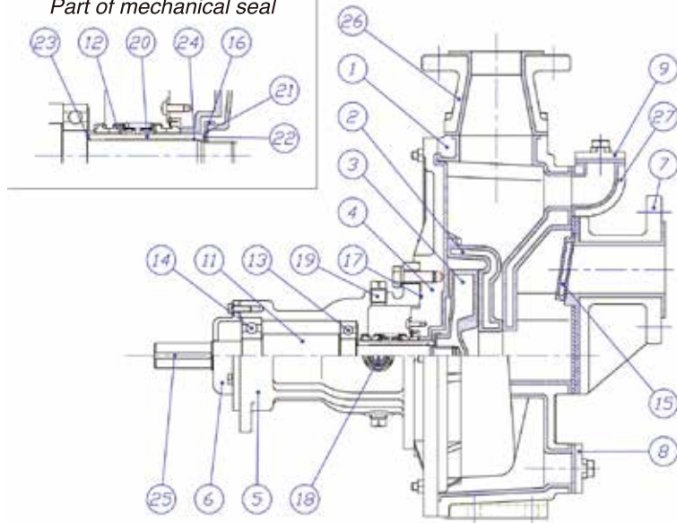
メカニカルシール部詳細 Part of mechanical seal
